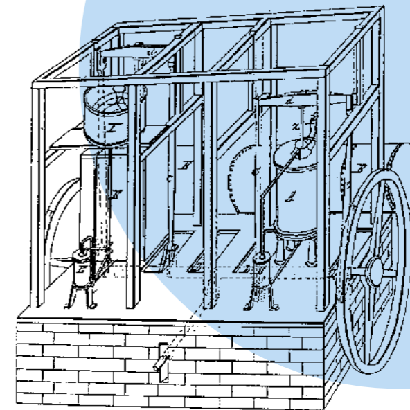
«Машина для производства льда» Джона Горри
